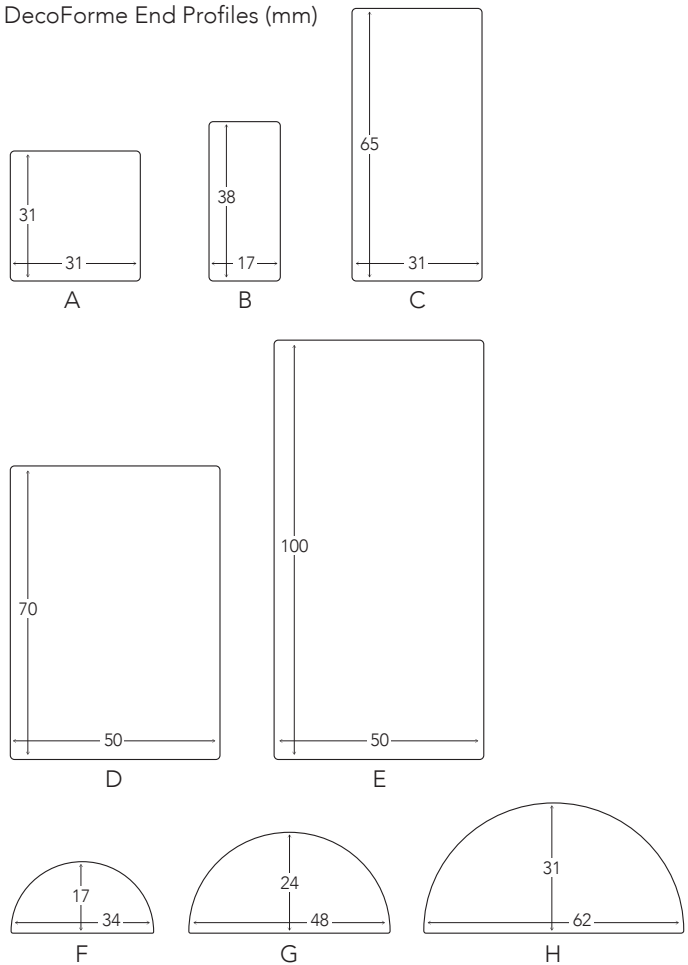
DecoForme End Profiles (mm)
